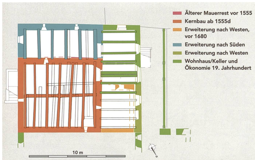
Kellergrundriss mit eingetragenen Bauphasen.
