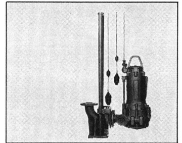
Fäkalien- Pumpen
