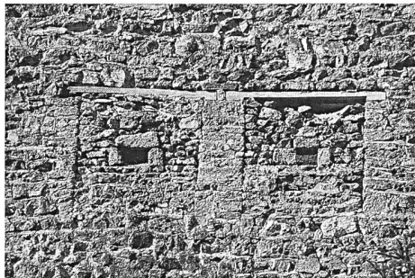
Abb. 134: Brienz/Brinzauls, Burgruine Belfort. Die nach- träglich zugemauerten Wehrfenster in der Nord- fassade.
