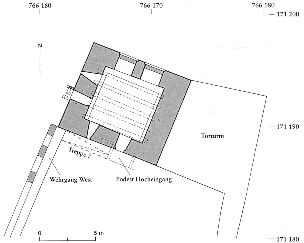
Abb. 141: Brienzen/Brinzauls, Burgruine Belfort. Grundriss drittes Geschoss. Mst. 1:200.
