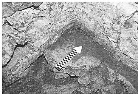
Abb. 142: Brienzen/Brinzauls, Burgruine Belfort. Rest des Mörtelbodens zum dritten Geschoss.
