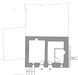
Kellergeschoss
