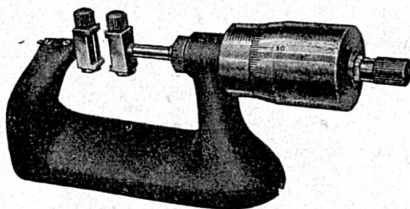
MICROMÈTRE pour mesurer les diamètres sur flancs des vis au moyen de 3 fils.
