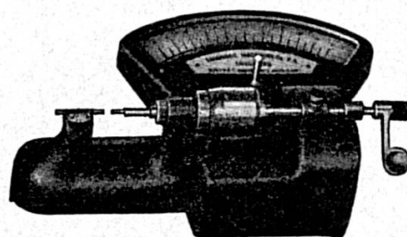
MICROMÈTRE- COMPARATEUR
