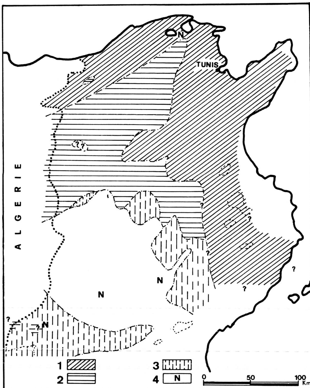
FIG. 6. — Distribution des faciès au cours de l'Eocène inférieur et du Lutétien inférieur en Tunisie d'après BUROLLET (1967).
