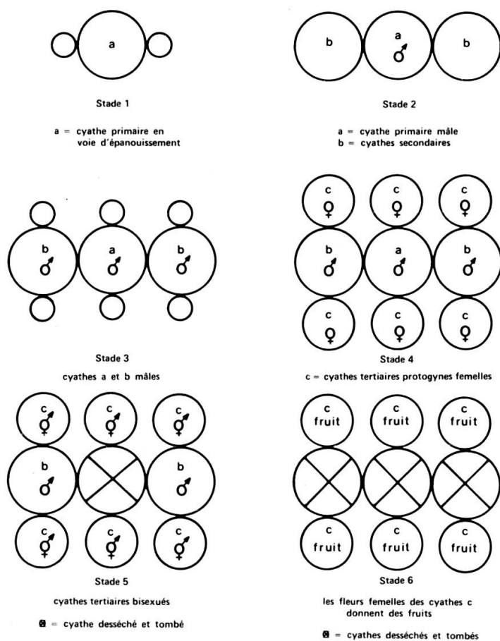
FIG. 6. — Déroutement de la floraison d' Euphorbia kamerunica .
