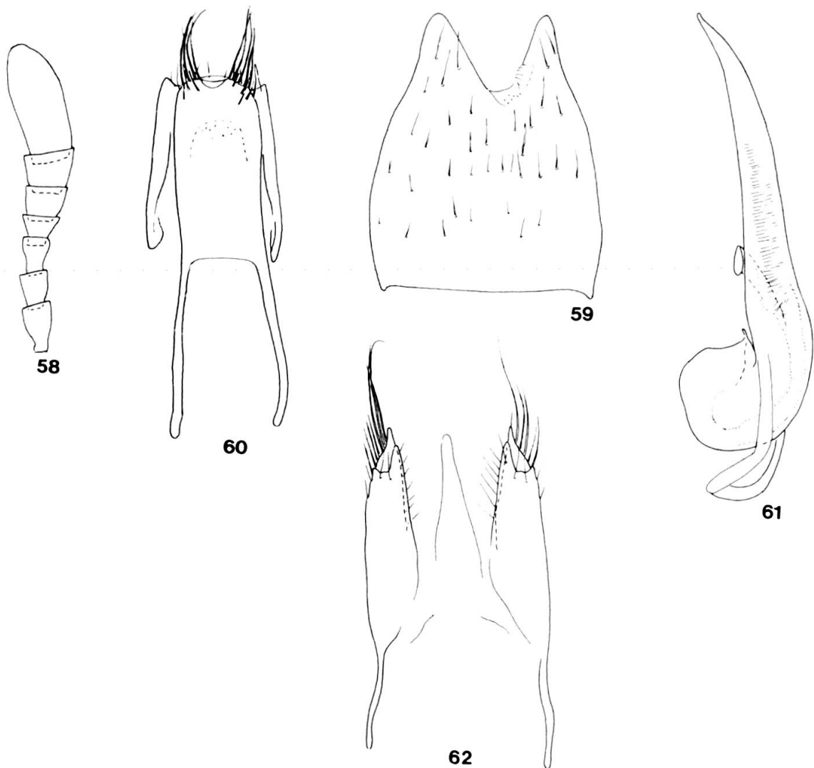
FIGS 58-62. H. hunanensis : 58, articles antennaires II à VIII; 59, sternite VI, mâle; 60, sternite VII, mâle; 61, édéage; 62, sternite génital, femelle.
