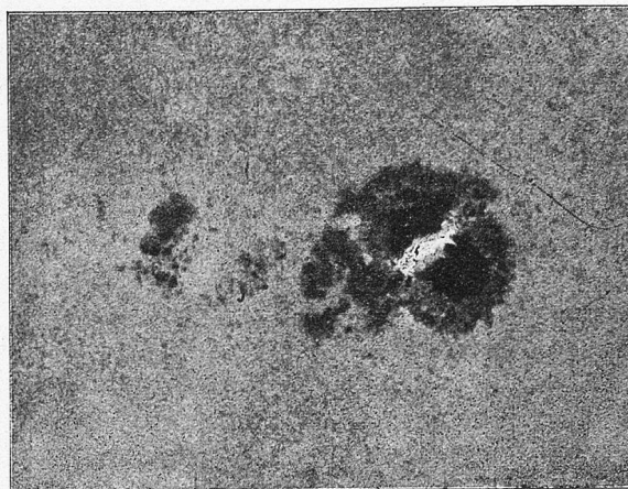
Große Sonnenfleckengruppe.
