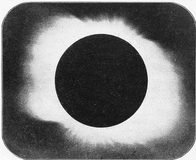
Die Sonnenkorona, aufgenommen während einer totalen Sonnenfinsternis am 28. Mai 1900 von Prof. Rijschey.
