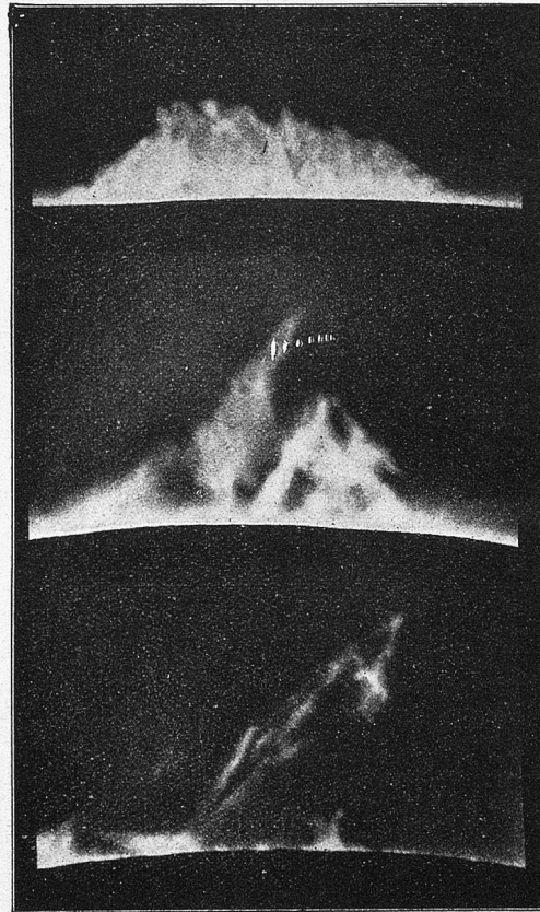
Veränderung einer Sonnenprotuberanz.
