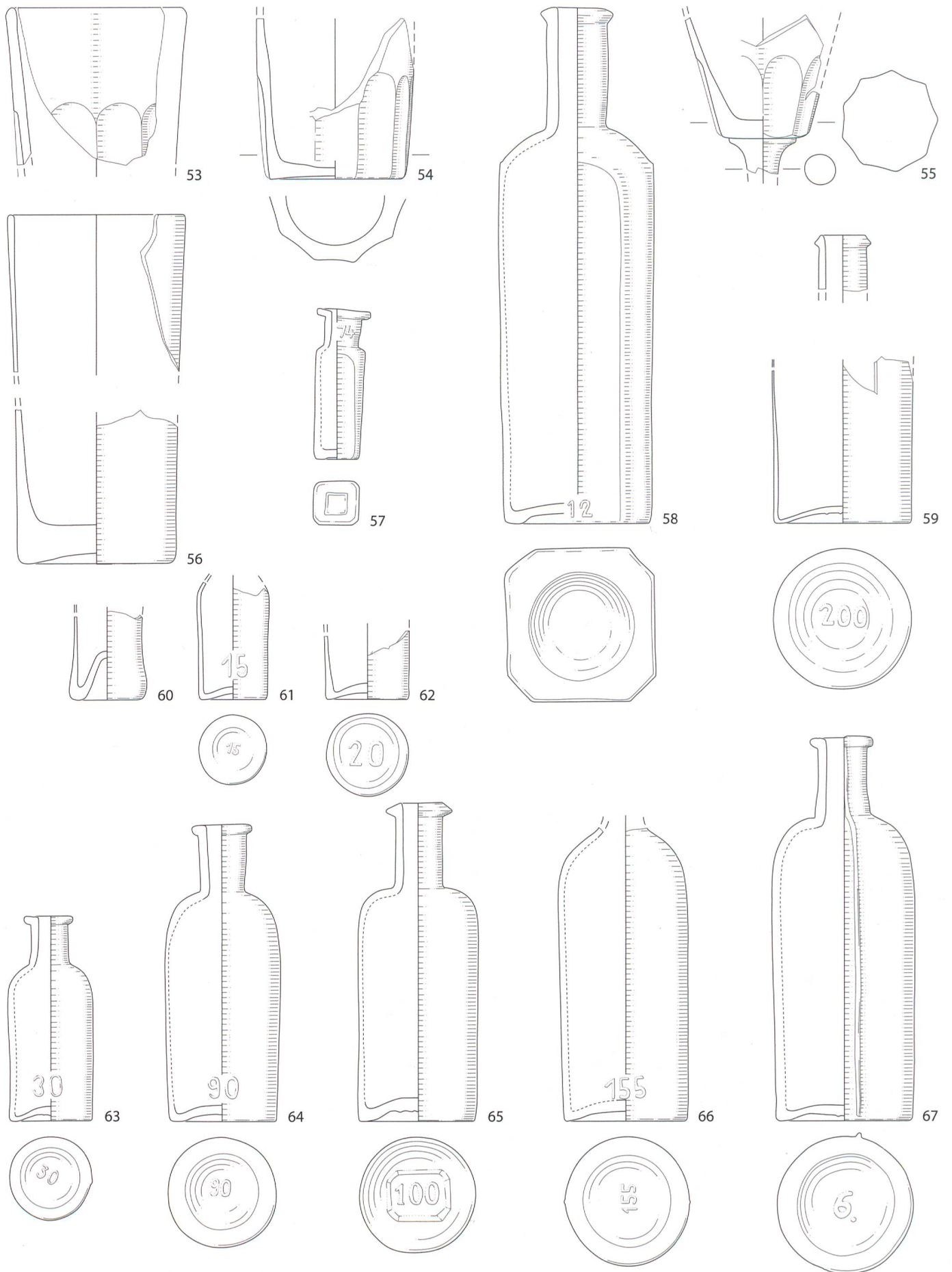
Abb. 14: Bern, Enghaldenstrasse 4. Glasfunde aus dem Latrinenschacht, um 1880/90 (vor 1892/1894). M. 1:2.
