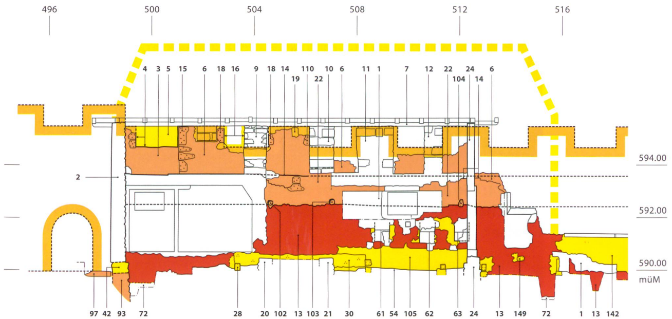
Abb. 3: Köniz, Schloss, Muhlenstrasse 15. Umzeichnung und Phasenplan der Nordmauer des Rossstalls, Südfassade. Phase 2 mit postuliertem Torturm in der Ringmauer. M. 1:150.
