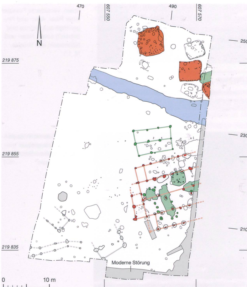
Abb. 1: Bätterkinder, Bahnhofstrasse 3. Eingetieftete Strukturen und identifizierbare Konstruktionen. Vorschlag zur chronologischen Stellung. Mittelalter: Phase 1 (grün) und 2 (rot), Phasen 1 bis 2 (blau). Neuzeitlich und modern (grau). M. 1:500.
