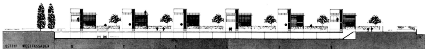
Längsschnitt / Ansicht, oben mit Tiefgarage
