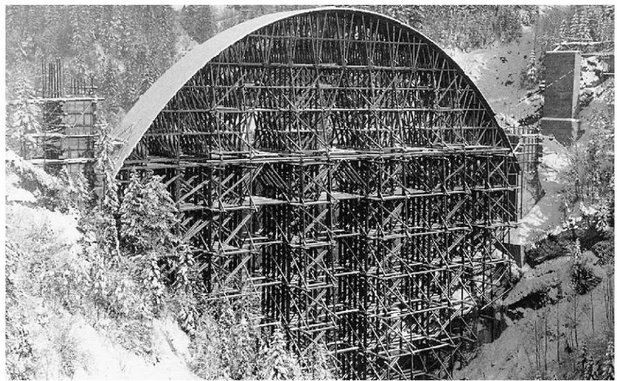
Das Lehrgerüst für die 79,6 m weit gespannte Hauptöffnung, Dezember 1907.
