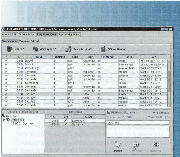
Illustration 4: affichage des commandes en cours et de leur statut
