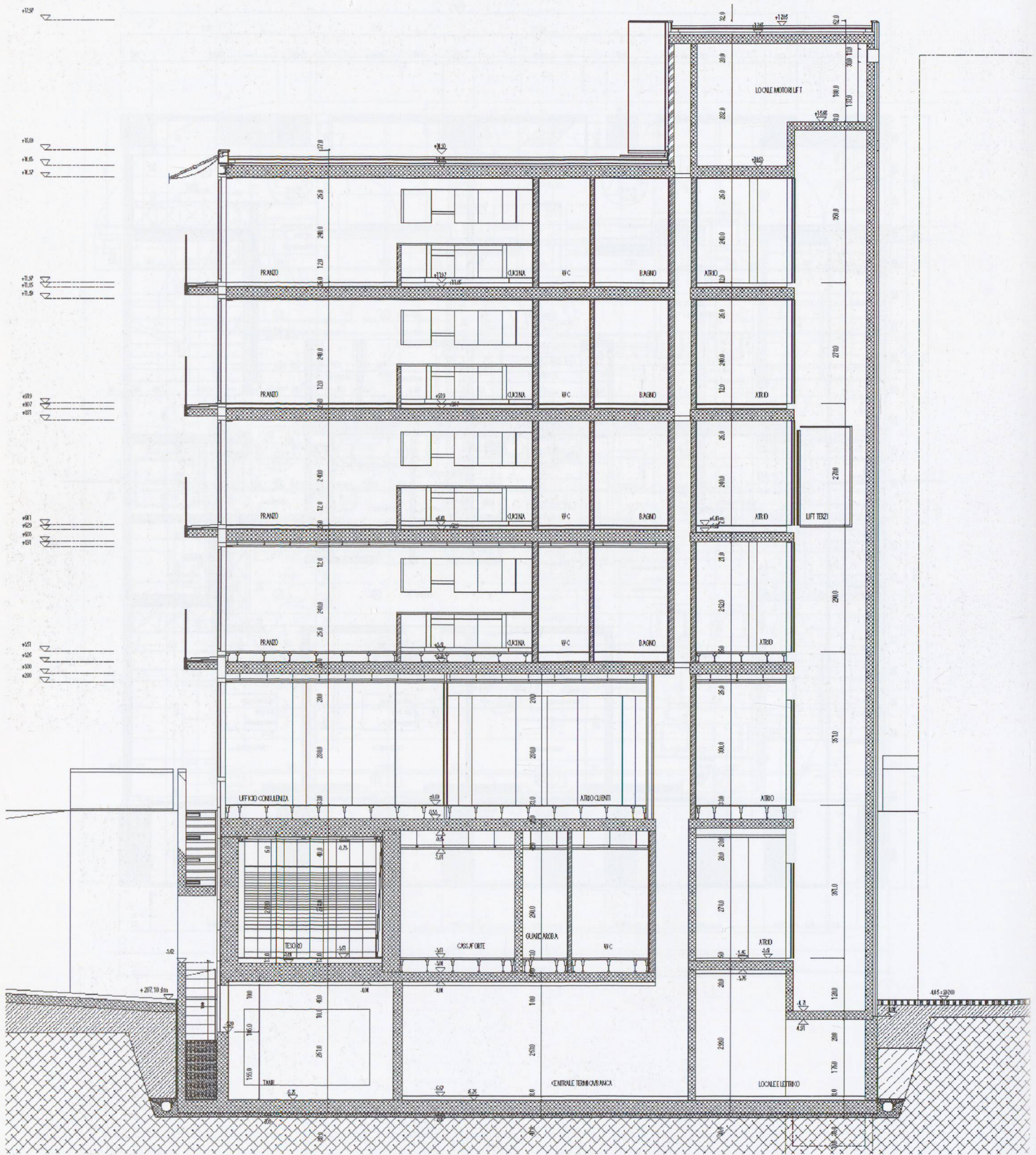
Sezione
