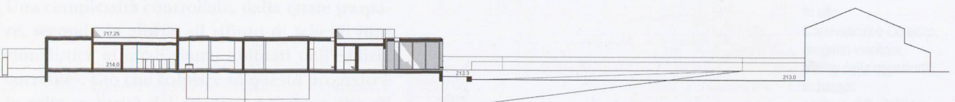
Sezione sud
