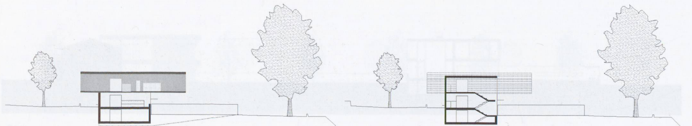
Sezioni
