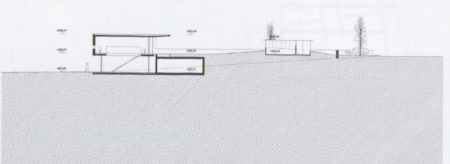
Sezione BB
