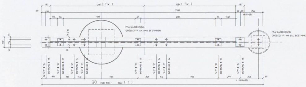
DRAUSICHT
