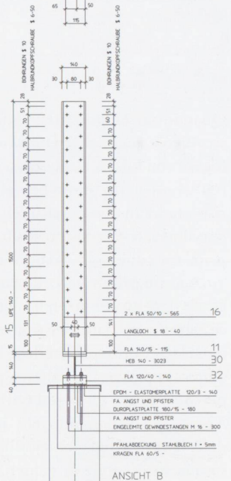
ANSICHT B
