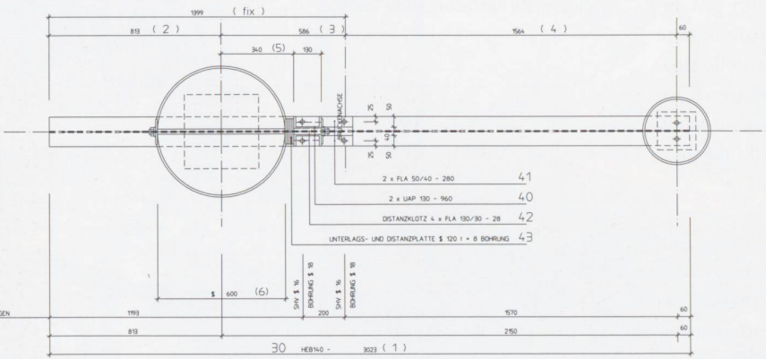
UNTERSICHT
