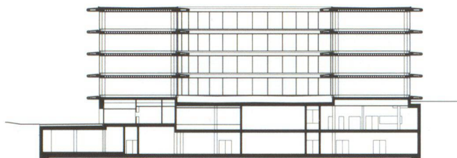
Sezione
