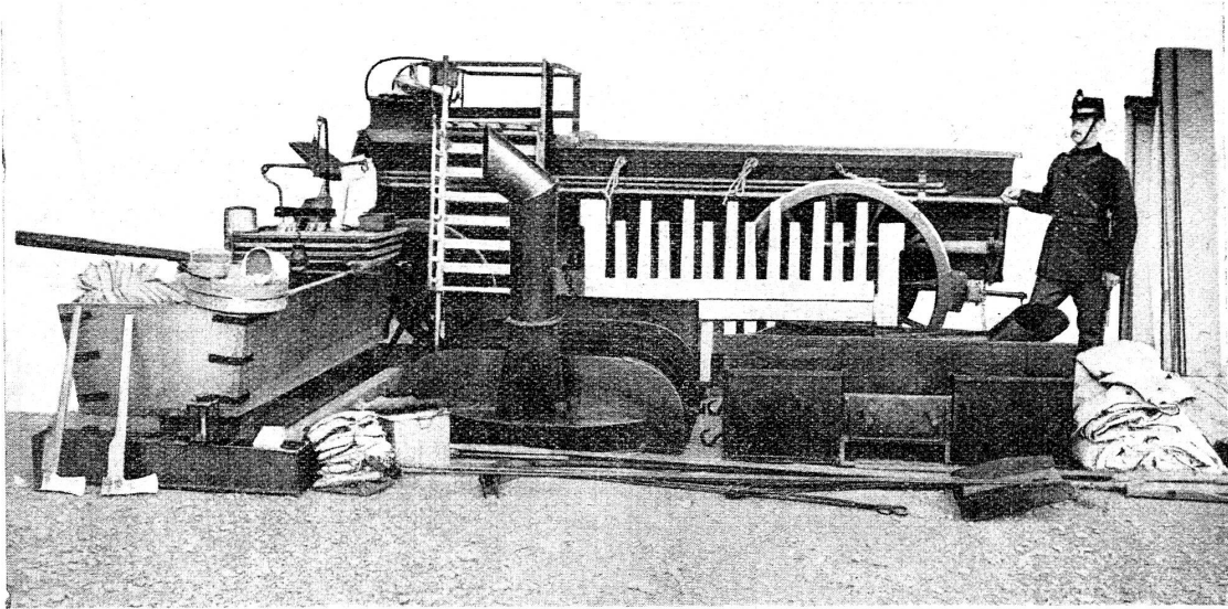
1885: Gerätschaftswagen abgeladen. Im Vordergrund die eisernen Ofenteile, links Backmulde und Bäckerei-Utensilien.
