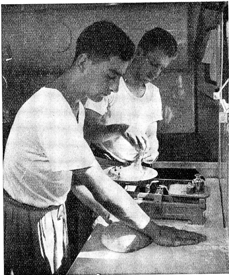
Mobile Bäckerei: Abwägen und Aufwirken der Teigbrote.
