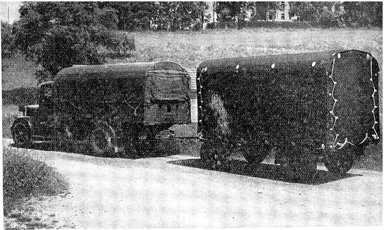
Mobile Mühle auf dem Transpo
