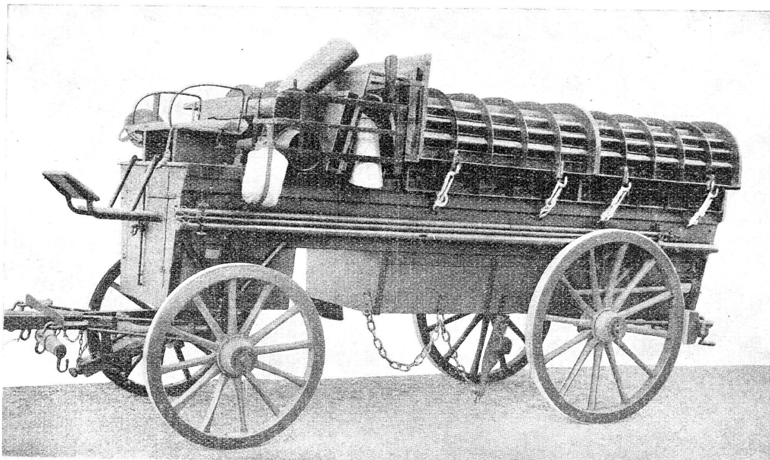
Gerätschaftswagen Ordonnanz 1885. Auf zwei solchen Gerätschaftswagen war eine Feldbäckereigarnitur verladen. Die gerippten Eisenteile wurden auf die Ofensohle aufgelegt und bildeten den Backherd.
