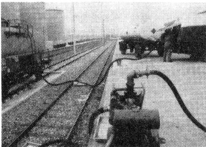
So sieht eine Betriebsstoffabgabestelle für Grossverbraucher aus.
