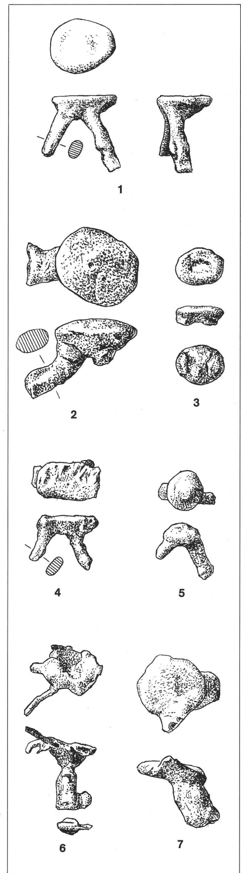
Abb. 12 Gussköpfe aus Bronze: 1-5 mit zwei, 6-7 mit einem Gusskanalzapfen. M. 2:3. Zeichnung O. Garraux. Restes de »l'étoile de fonte«. Boccamì.
