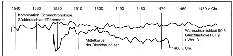
Abb. 15 Deckungslage der Jahringkurve der Blockhölzer auf dem Kombinationsmittel aus der süddeutschen Eichen- und der dänischen Baumsargchronologie. Recouplement de la courbe dendrochronologique des bois du blockbau avec la moyenne combinée des cercueils en troncs de
