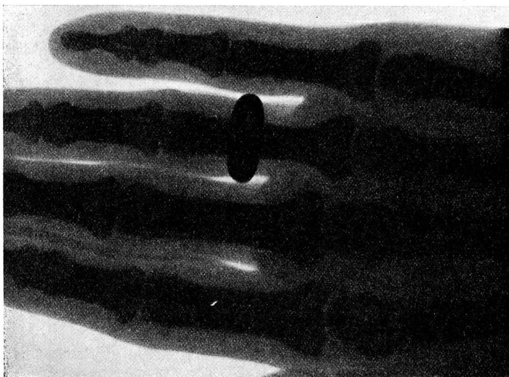
Figure 29. Autotypie d'une radiographie due à des rayons X engendrés dans une ampoule radiogène par la haute tension asymétrique d'un transformateur de \frac{100}{100\,000} volts. (Sa reproduction ne rend pas les nuances du négatif radiographique.)
