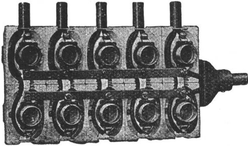
Abb. 16. Uzedgruppe mit eingelegten Abzwegleitungen und aufgelegter Sammelschiene.
