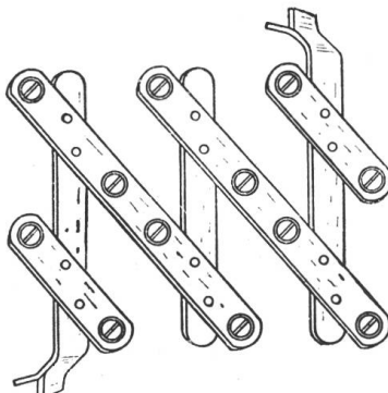
Abb. 19. Mehrfach Dübel für ältere Universalversicherungen.
