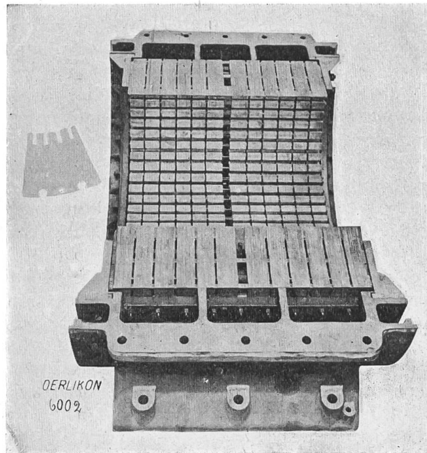
Fig. 5. Luftführung im Stator eines Turbogenerators. Maschinenfabrik Oerlikon.
