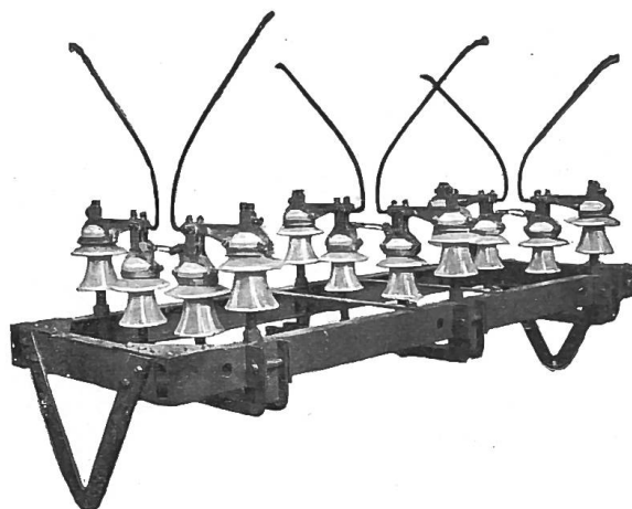
Abb. 29. Ausschaltbare Freileitungs-Sicherung der A.-G. Sprecher & Schuh.
