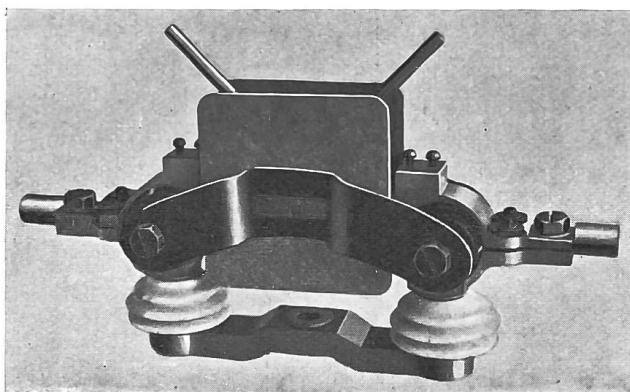
Abb. 34. Sicherung mit magnet. Funkenlöschung der A.-G. Sprecher & Schuh.
