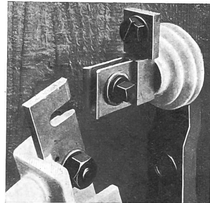
Abb. 8. Klemmkontakt für grössere Stromstärken.
