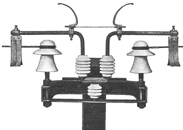
Abb. 30. Aushängbare Freileitungs-Sicherung der A.-G. Sprecher & Schuh.
