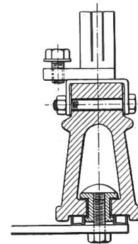
Abb. 21. Aufgeklemtte Kontakt- und Befestigungsteile der Hochsp.-Sicherung der A.-G. Sprecher & Schuh.
