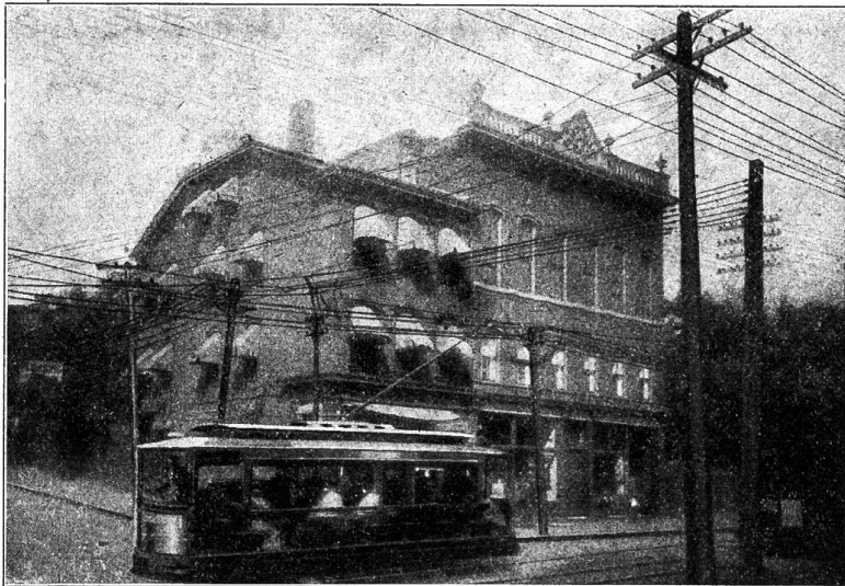
Fig. 3 zur Fussnote Seite 279. Hochspannungs- und Telefon- und schwere Niederspannungs-Freileitungen in Pittsburg Pa.
