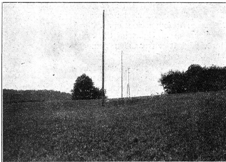
Abb. 2. Schablonenhaft durch einen Waldrand geschlagene Schneise. Die links stehen gelassene Baumreihe hätte zum Mindesten entfernt werden sollen. Leitung im Baustadium.
