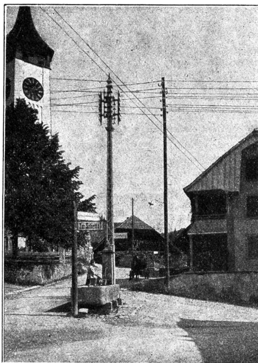
Abb. 6. Unbefriedigende Aufstellung von Masten. Der Gitterträger steht im Kreuzungspunkte zweier Strassen und die hinterste Stange im Gabelungspunkt einer Strasse.
