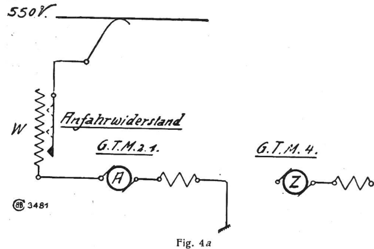
Schaltung bei Fahrt auf der Adhäsionsstrecke (vorwärts bzw. rückwärts).
