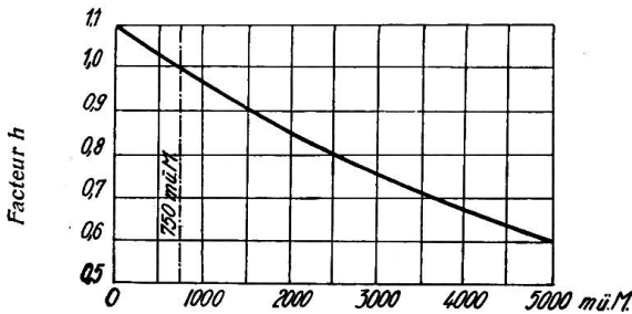
Fig. 2. Facteur h en fonction de l'altitude.
