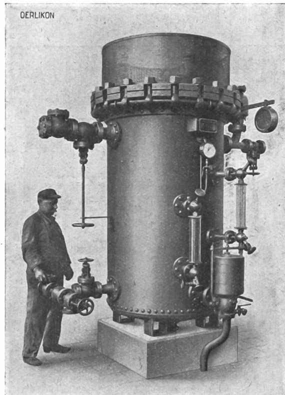
Fig. 5. Hochspannungs-Elektrodenkessel.
