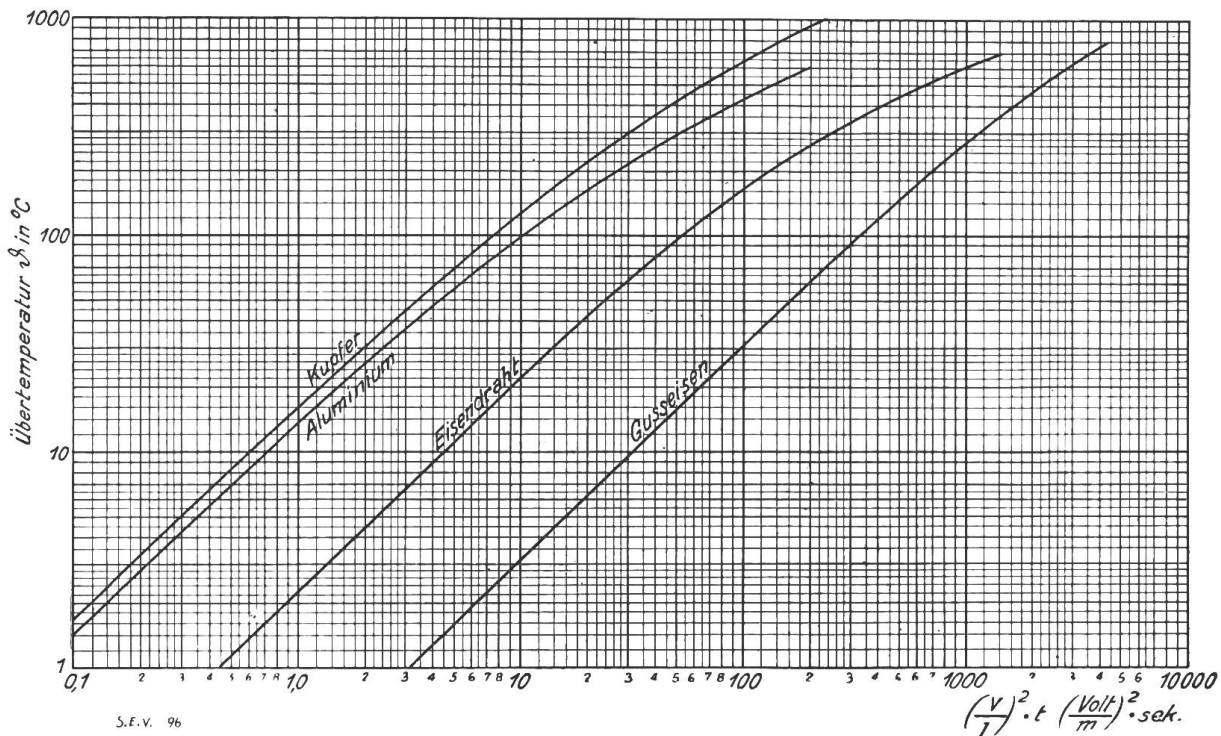
Fig. 7. Kurven zur Ermittlung der Uebertemperatur von verschiedenen Leitermaterialien bei kurzzeitiger ohmscher Belastung mit konstanter Spannung.
