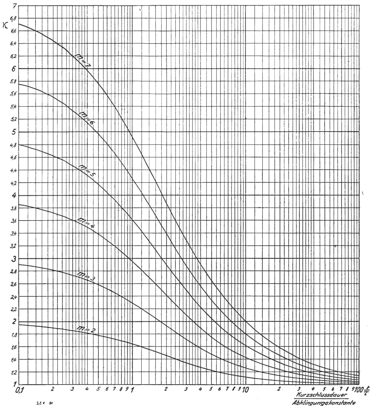
Fig. 5. Korrekturfaktor \alpha zur Berücksichtigung des Abklingens des Kurzschlussstromes.
