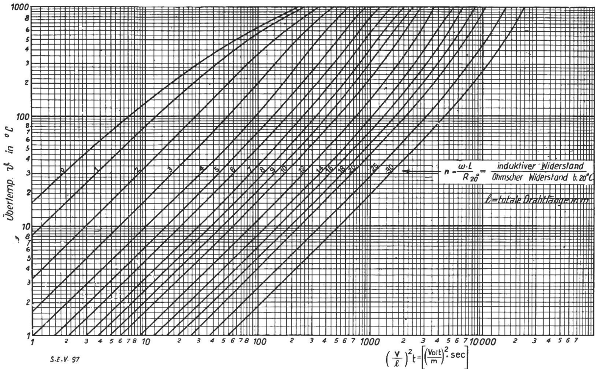
Fig. 8. Kurven zur Ermittlung der Uebertemperatur von Spulen aus Cu-Draht bei kurzzeitiger induktiver Belastung und konstanter Spannung. Ausgangstemperatur = 20° C. ( \rho für Cu, bei 20° C = 0,0175 \Omega /m u. mm 2 ).
