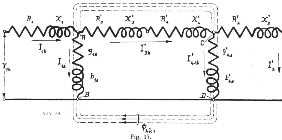
Ersatzschaltung beim Kurzschlusszustand bei Primärspannung.
