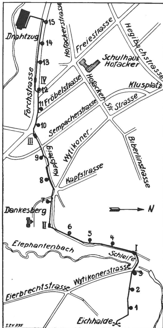
Fig. 3. Lageplan der Kabelleitungen Eichhalde-Drahtzug 1 : 10 000. ● 1 bis 15 Temperatur-Messstellen. ■ I bis IV Muffenschächte.
