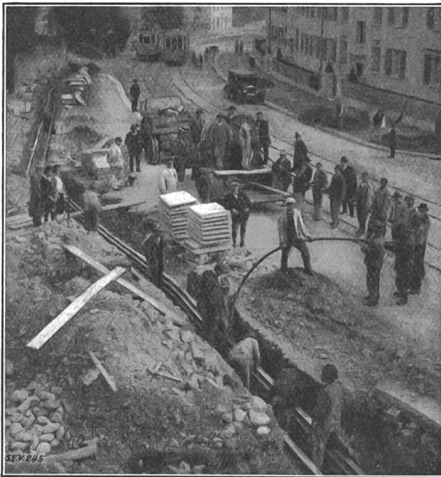
Fig. 13. Auslegen des Kabels von der Trommel in den Kanal. (Forchstrasse, 20. Oktober 1926).
