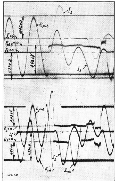
Fig. 9. Begünstigung des Abschaltvorganges durch asymmetrischen Stromverlauf. Der Lichtbogen der Phase I löscht bei ersterem um 90^\circ phasenverschobenem Nulldurchgang, um nach 0,013 sec. wieder zu zünden. Die endgültige Löschung erfolgt dann nach weitem 0,02 sec.
