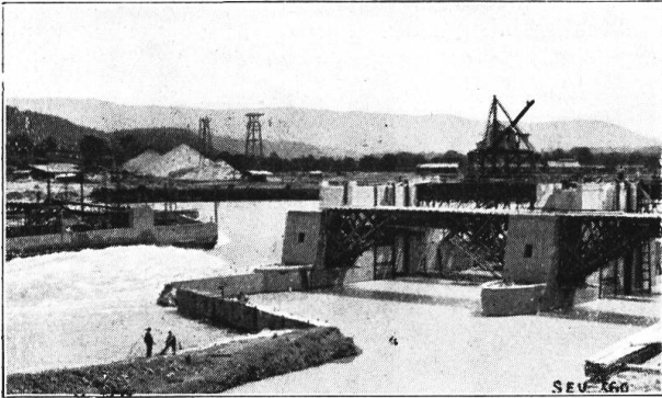
Baustelle Ryburg-Schwörstadt.
