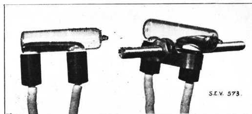
Fig. 4. Quecksilberkontakt für Relais (Brown, Boveri).
