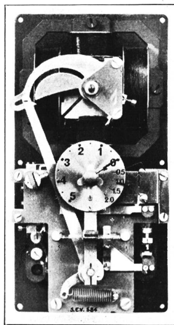
Fig. 14. Brown, Boveri-Distanzrelais. Vorderansicht. Ruhestellung.
