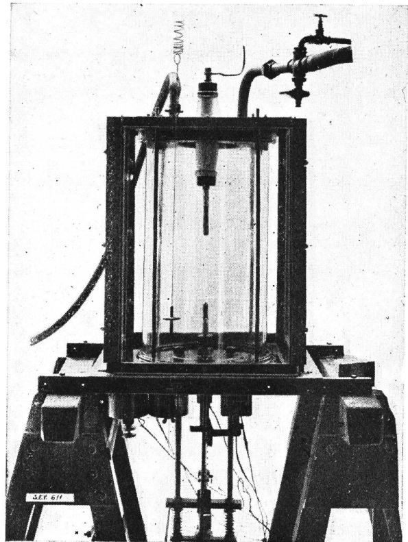
Fig. 19. Oelschalter für Aufnahmen mit der Zeitlupe. Der Schalter besteht aus einem Glaszylinder und einem rechteckigen Glaskasten. Oelvolumen ca. 90 Liter.
