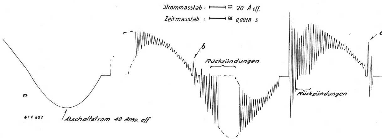
Fig. 17. Einfluss von Parallelkapazitäten zu Oelschaltern auf den Abschaltvorgang. C = 0,177 \cdot 10^{-6} F . Kathodenoszillogramm des Kurzschlussstromes in D. Kapazität angeschlossen vor der Drosselspule. (Fig. 17 a.)
