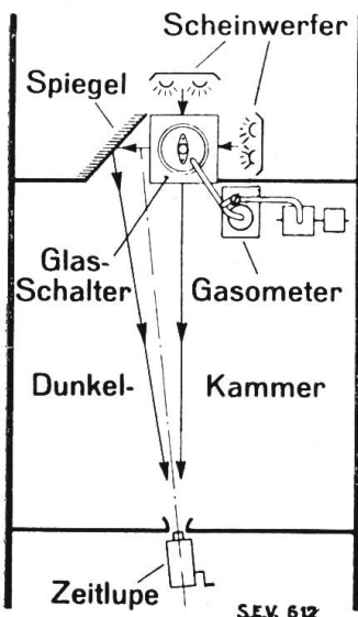
Fig. 20. Grundriss der Versuchsanordnung für Zeitlupenaufnahmen. Bis 300 Bilder/sec.
