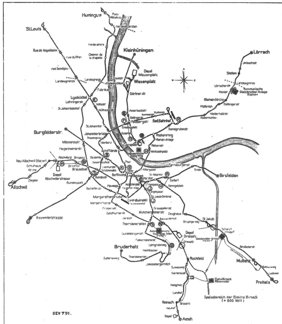
Fig. 1. Uebersichtsplan der Stromverteilung.
