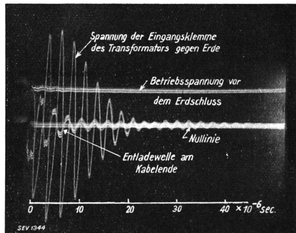
Fig. 34. Entladungswellenresonanz.
