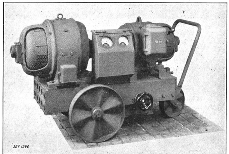
Fig. 2. Schweissmaschine der A.-G. Brown, Boveri & Co.
