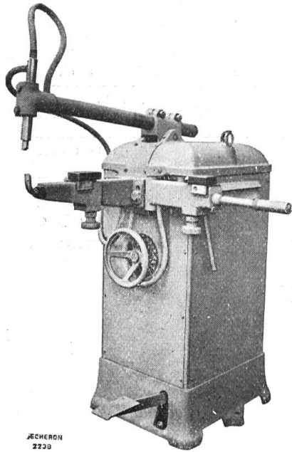
Fig. 1. Universalschweißmaschine der S. A. des Ateliers de Sécheron.
