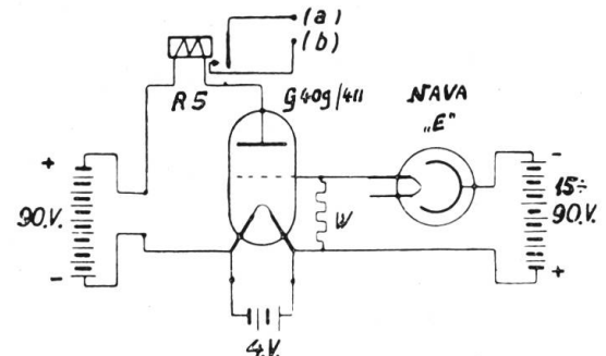
Fig. 4. Einfachste Schaltung eines „Lichtrelais“ (1 Zelle Nava „E“, 1 Rohr G 409 oder 411, 1 Relais R 5 und Hilfsbatterien.)
