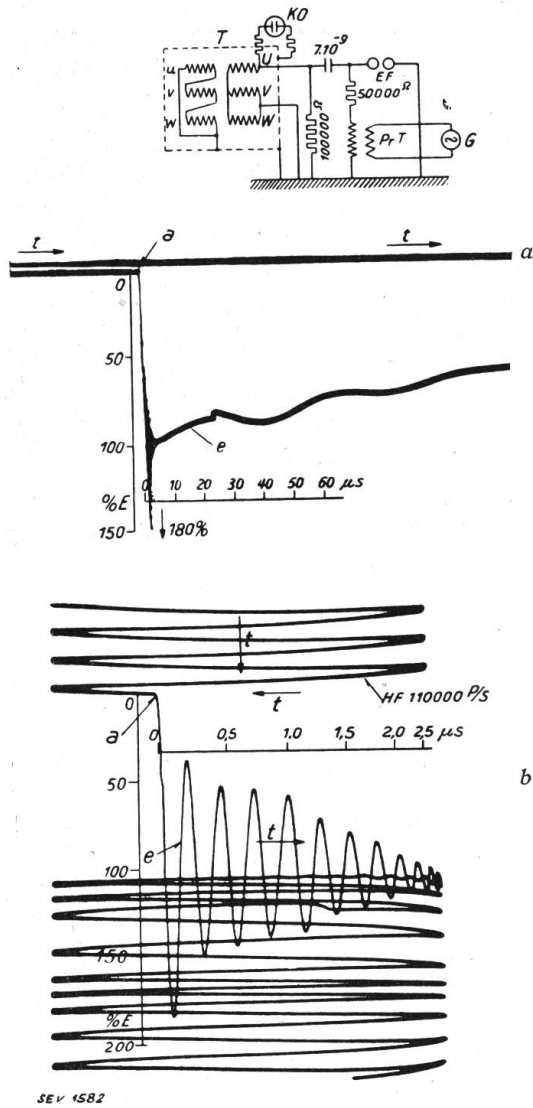
Fig. 13. Kathodenstrahloszillogramm der Spannung zwischen Klemme U und Erde bei Stossprüfung nach Fig. 3. Ueberschwingen der Klemmenspannung bis 180\% E . C = 7 \cdot 10^{-9} F, R = 100\ 000 Ohm, r = 50\ 000 Ohm. Pr.T = Prüftransformator. Hochfrequenzschwingung mit f = 4,2 \cdot 10^6 Per/s.
