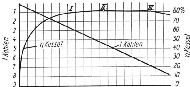
Fig. 4. Belastungskurve eines Eisenbahnkraftwerkes, komb. Projekt Riley Stoker und Speicher.
