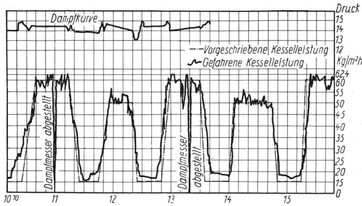
Fig. 3. Versuch über Anpassungsfähigkeit an Belastungsschwankungen, gefahren am 20. Mai 1929 im Kreiskraftwerk Spandau. Kesselgrösse 940 m 2 , 15 atü.
