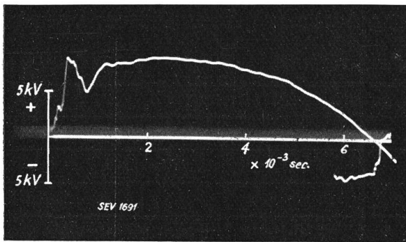
Fig. 12. (f) Versuchs-No. 314; Messung in Phase: 3 (Leitungsseite des Induktionsreglers).
