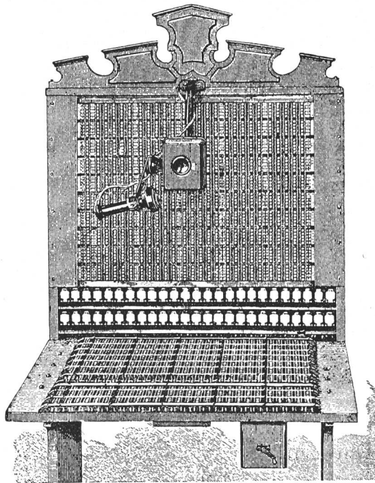
Fig. 4. Erste Umschaltvorrichtung.
