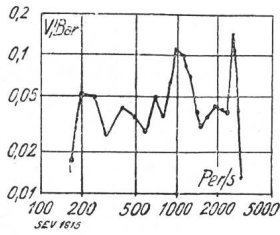
Fig. 6. Frequenzkurve eines normalen Fernsprechmikrophons.
