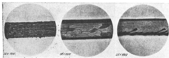
Fig. 1. Nach dem Hämmerverfahren hergestellter Wolframdraht (Ziehstruktur).
