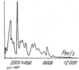
Fig. 8. Tonspektrum des Geräusches eines Staubsaugers (nach Grützmaier). Schalleistung in Funktion der Frequenz.
