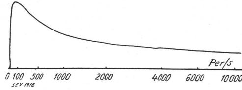
Fig. 7. Frequenzkurve eines Kondensatormikrophons.
