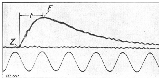
Fig. 22. Verlauf des Druckes bei einer Sprengstoffexplosion in der Löschkammer eines Oelschalters. Z Moment der Zündung. E Ende der Verbrennung. t Dauer der Verbrennung = 0,017 s. Druck im Moment E = 53,5 kg/cm 2 .
