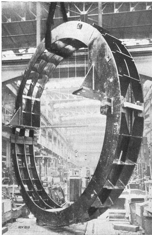
Fig. 8. Geschweisste Innenstator-konstruktion. (Sécheron).
