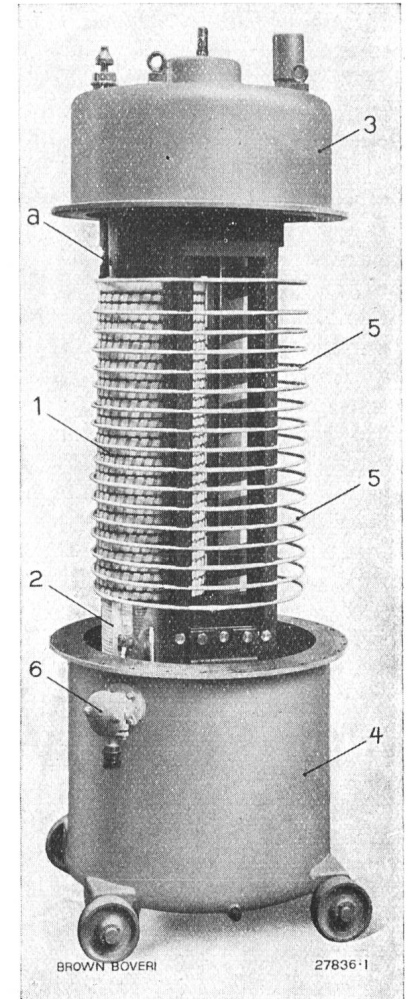
Fig. 23. Isoliermantel-Spannungswandler für hohe Spannungen. Isoliermantel abgehoben. (BBC.)
