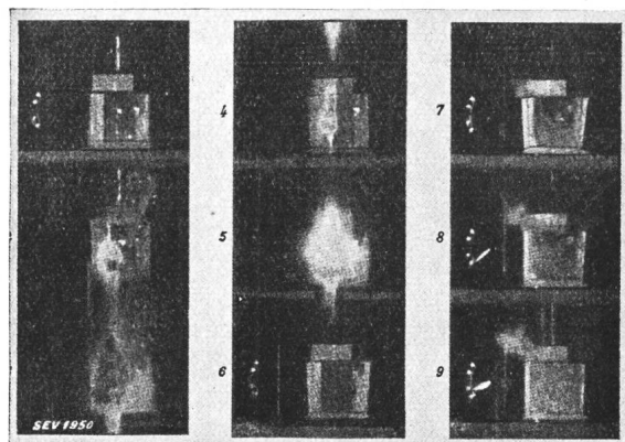
Fig. 32. Zeitlupenaufnahme einer Lichtbogenlöschung bei Bersten der Expansionskammer aus Glas.
