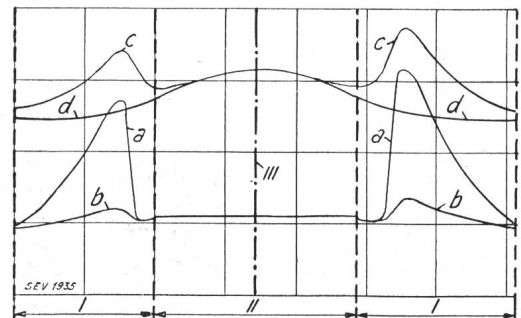
Fig. 9. Verlustverteilung und Erwärmung über einer Statorspule. (Aufnahme MFO).
