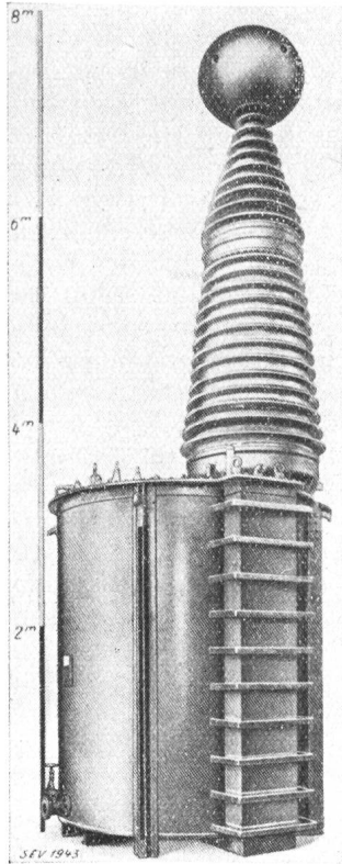
Fig. 21. Prüftransformator für 1000 kVA, 1 000 000 V. (AEG.)
