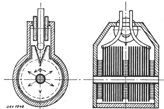
Fig. 27. Schema des Deïon-Schalters.
