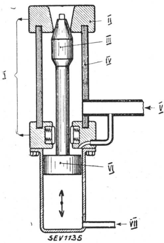
Fig. 30. Pressluftschalter. I Elektrischer Anschluss. II Fester Kontakt. III Beweglicher Kontakt. IV Isolationsmaterial. V Pressluftzufuhr zur Ausschaltung. VI Kontaktantrieb. VII Pressluftzufuhr zur Einschaltung.
