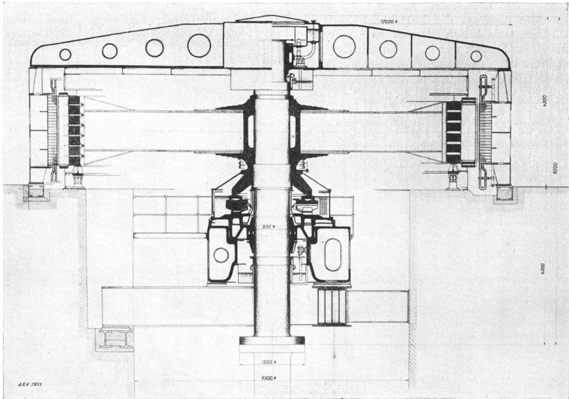
Fig. 7. Generatoren für die Beauharnois Power Corp. 75 U/m; 44000 kVA, 25 p/s (rechts), resp. 47000 kVA, 60 p/s (links). (MFO).
