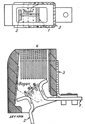
Fig. 28. Deïon-Motorschalter. 1 fester Kontakt. 2 beweglicher Kontakt. 3 Eisenjoch. 4 Platten.
