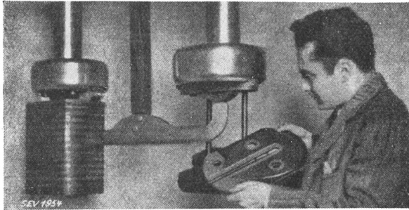
Fig. 29. Deion-Hochspannungs-Oelschalter. Kontakte für 110 kV.
