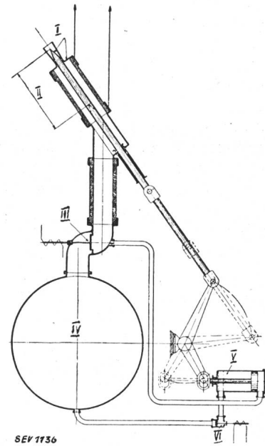
Fig. 31. Schematische Darstellung des Pressluftschalters für 15 kV Betriebsspannung.
