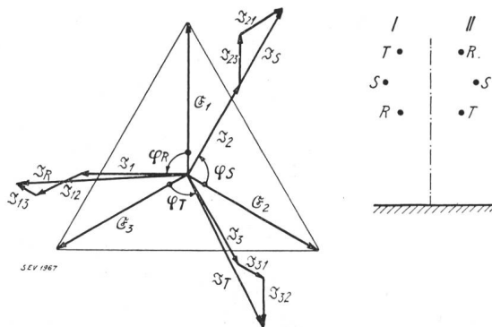
Fig. 6. Diagramm der leerlaufenden Leitung. Strang I. Rechts: Schema des Mastbildes. U_1, U_2, U_3 Phasenspannungen. I, S, T Leiterströme; diese setzen sich zusammen aus den Teilströmen I_1, I_2 und I_3 etc. Phasenspannung und Leiterstrom sind gegeneinander verschoben, und zwar um mehr als 90^\circ in Phase R, um 90^\circ in Phase S und um weniger als 90^\circ in Phase T.
